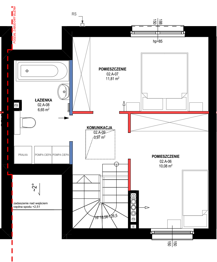
RZUT 1 PIĘTRA
