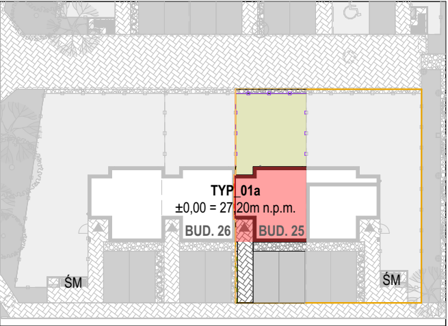
ZAGOSPODAROWANIE TERENU
