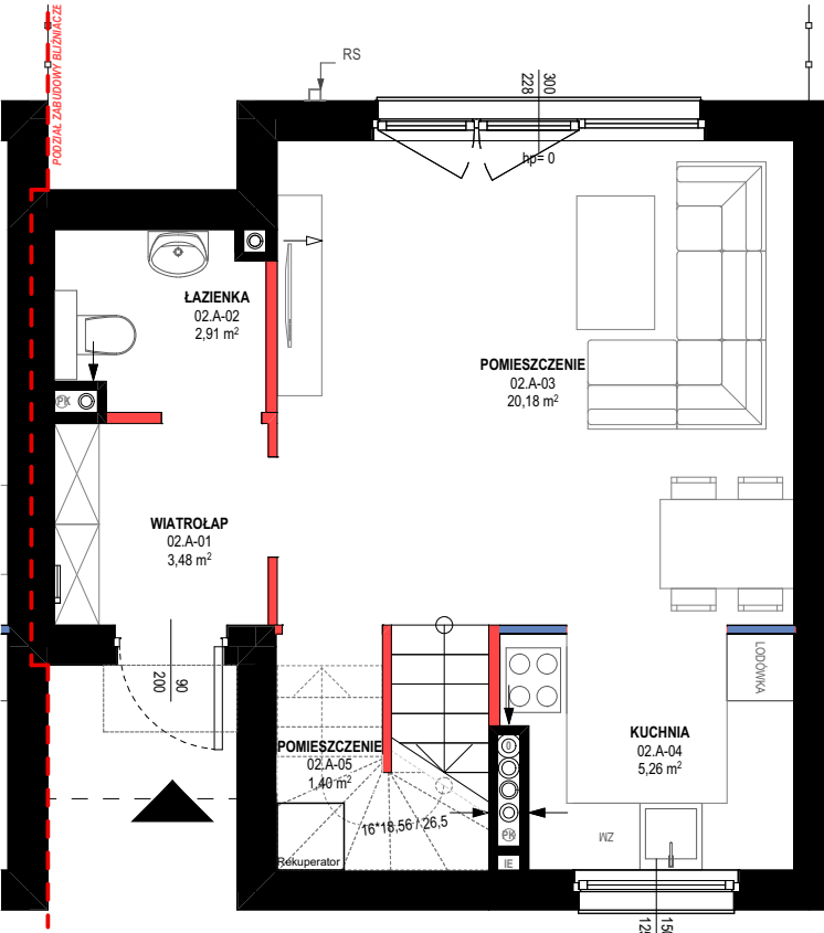
RZUT PARTERU
